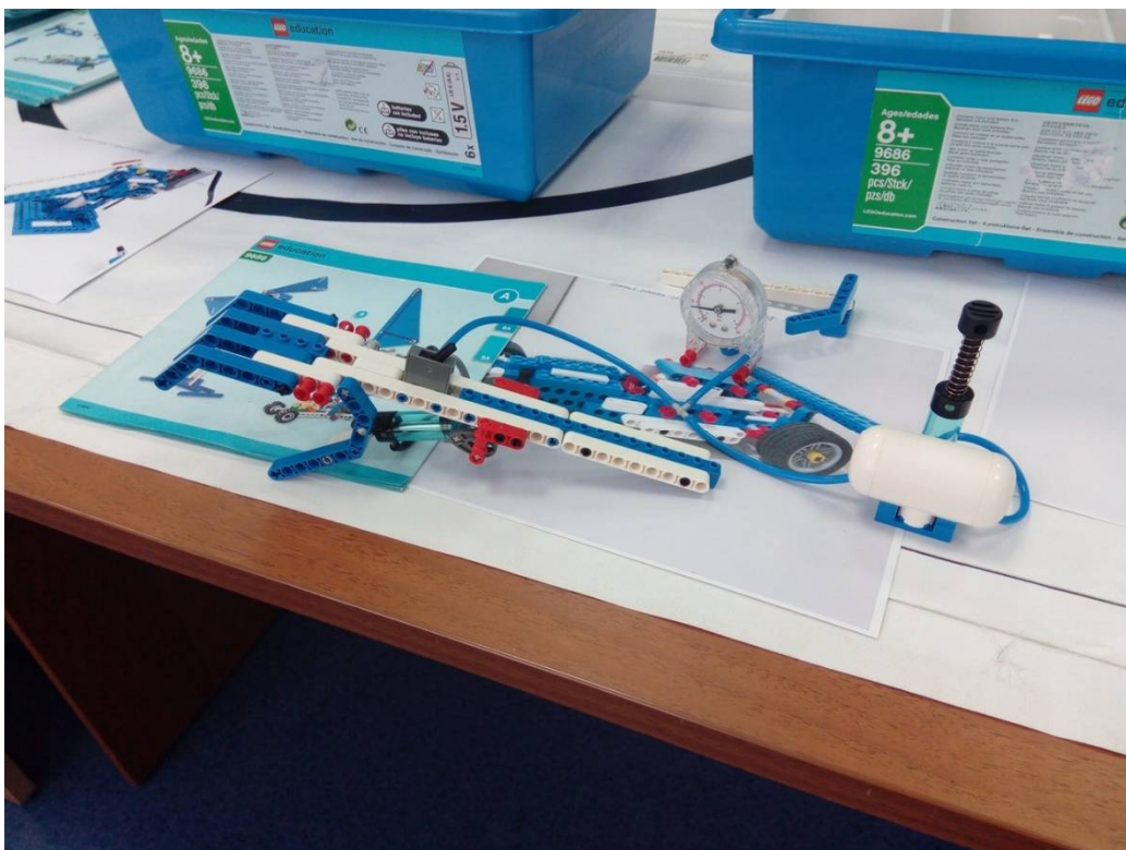
Пневматич. «мех.рука»
